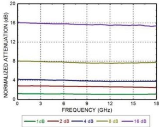
Attenuation
