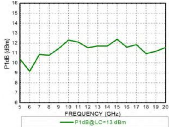
Input P1dB
